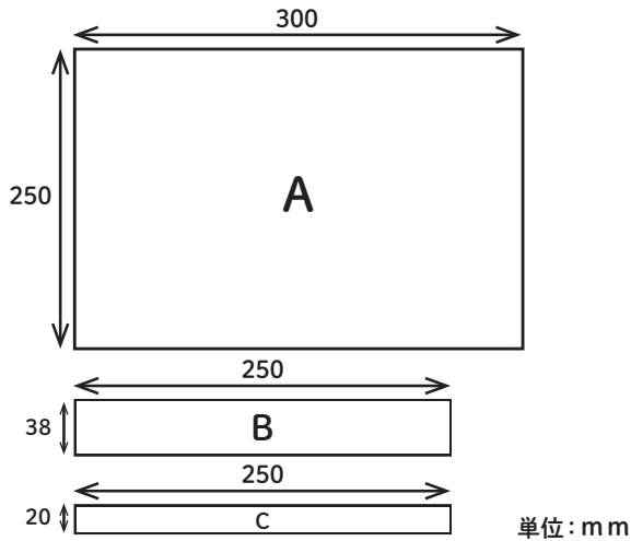
木取り図
