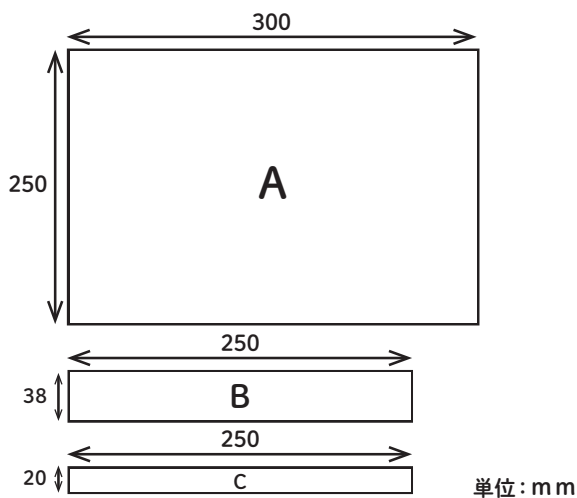
木取り図
